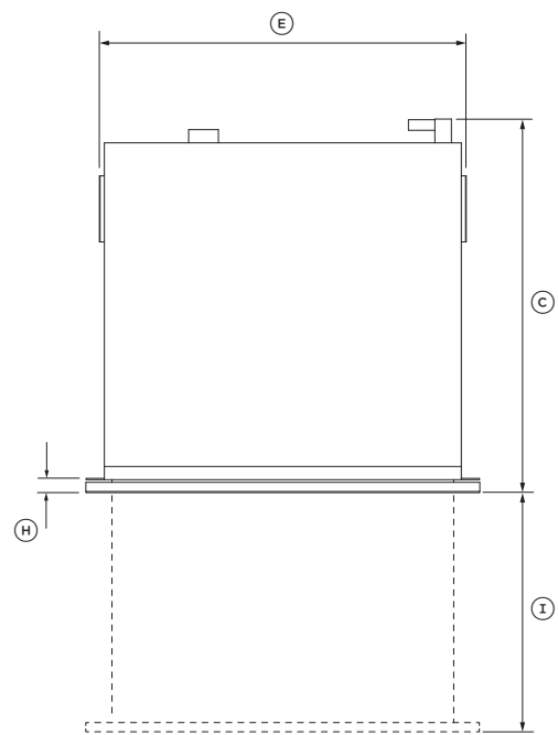
俯视图
